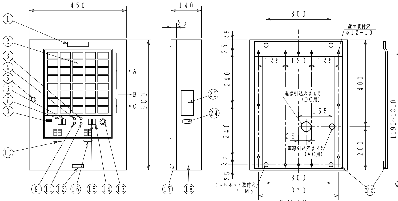
取付寸法図
