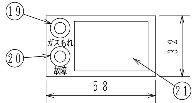
地区灯詳細図
