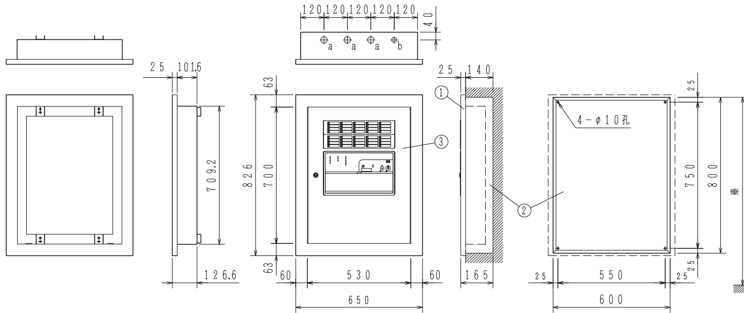
埋込枠 取付寸法詳細図 (正面図) ZBFJ004-B1
