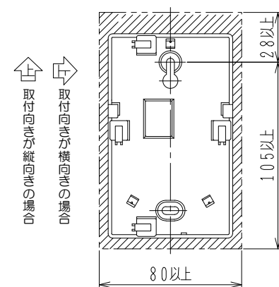
【取付ベースの取付寸法】
