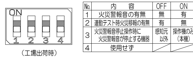
⑧ 機能設定スイッチ
