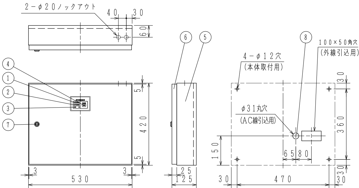
取付寸法図
