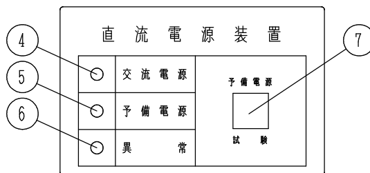
操作部詳細図
