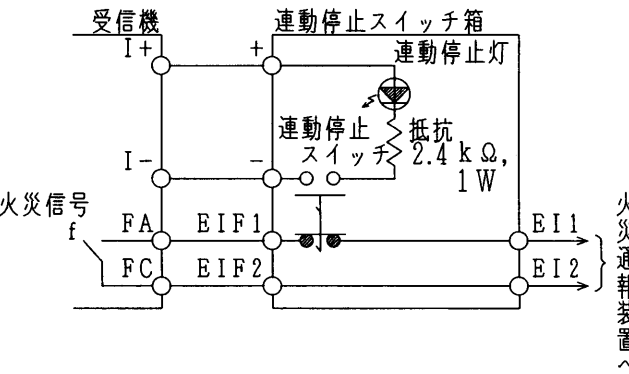
接続図
