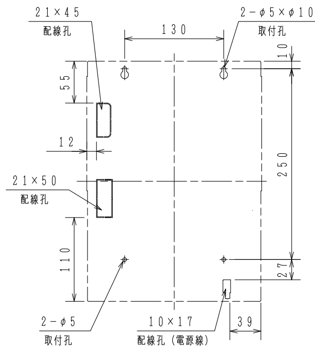
取付寸法図
