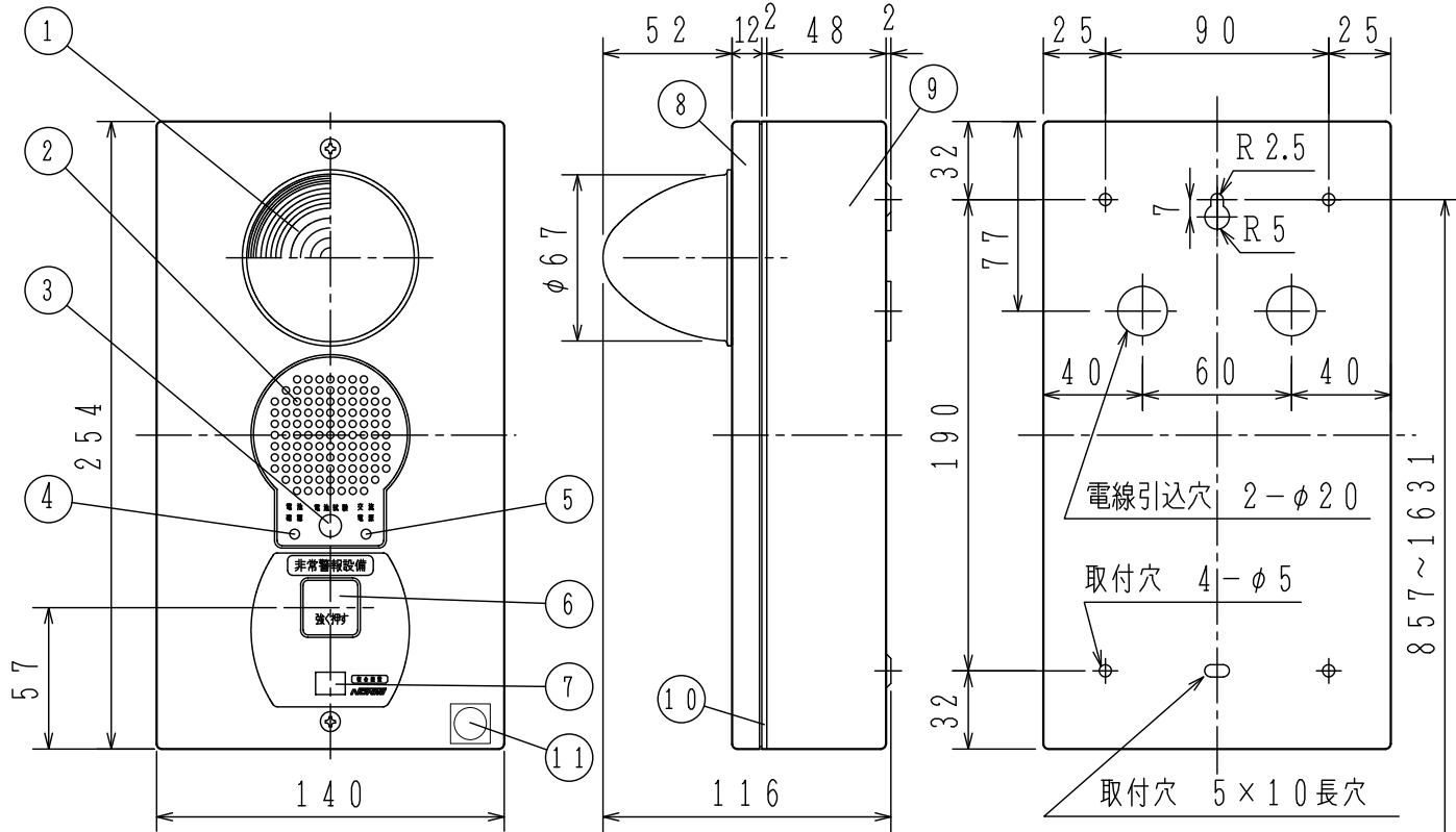
取付寸法図
