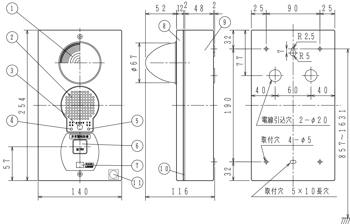
取付寸法図
