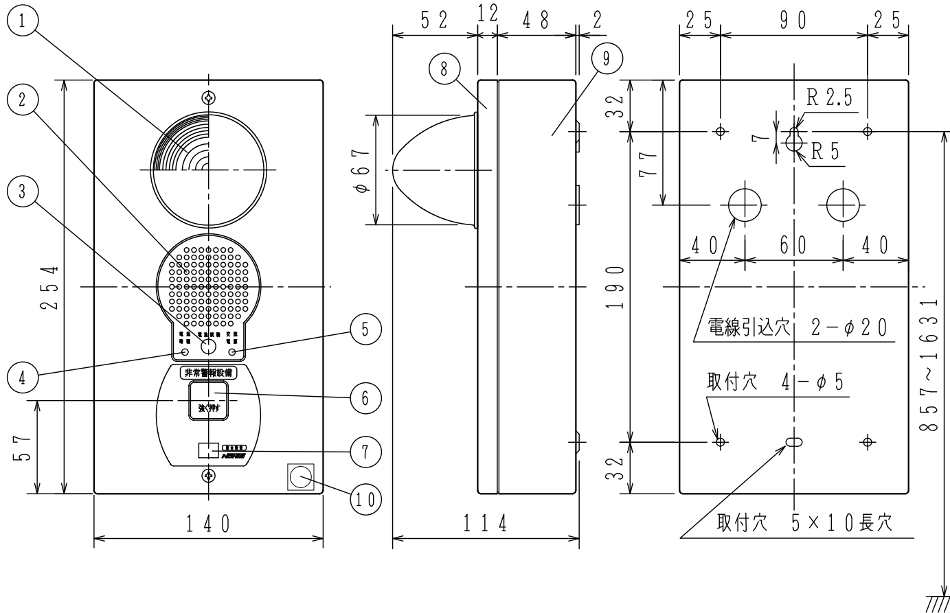
取付寸法図
