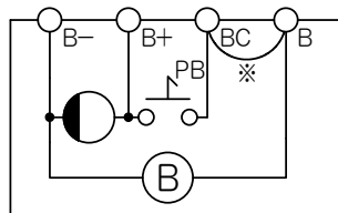
回路図
