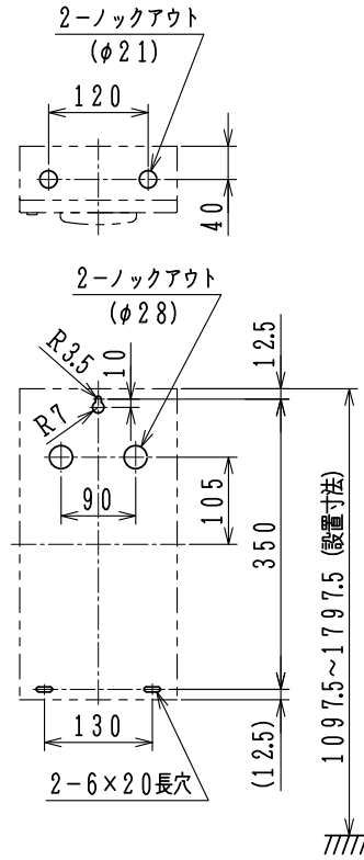
取付寸法図 (正面)
