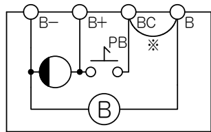
回路図
