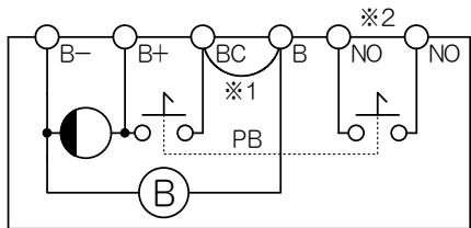
回路図
