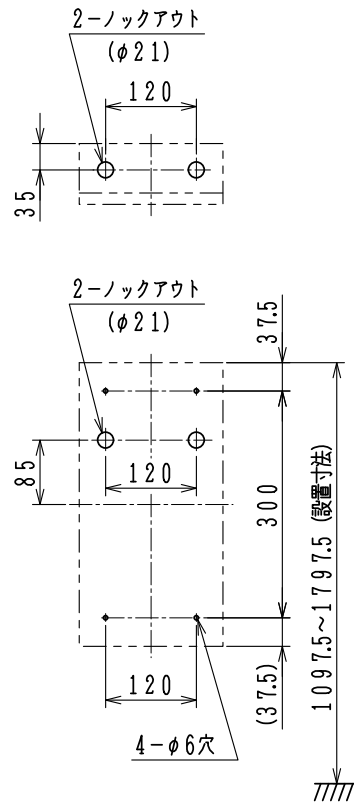
取付寸法図 (正面)
