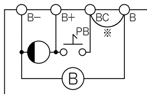
回路図
