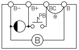
回路図
