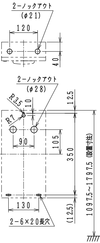
取付寸法図（正面）
