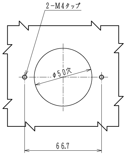
板金加工図
