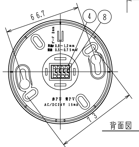
埋込ボックス使用の場合
