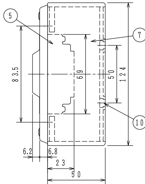
露出ボックス取付図
