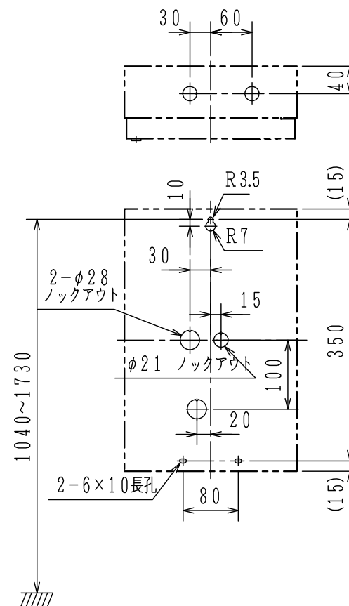
取付寸法図（正面）
