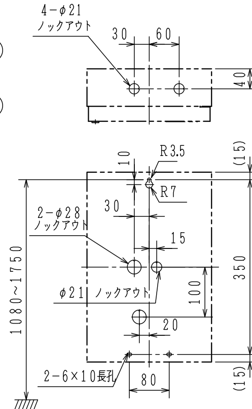
取付寸法図 (正面)
