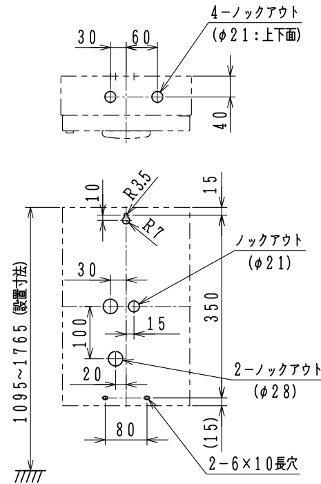
取付寸法図 (正面)
