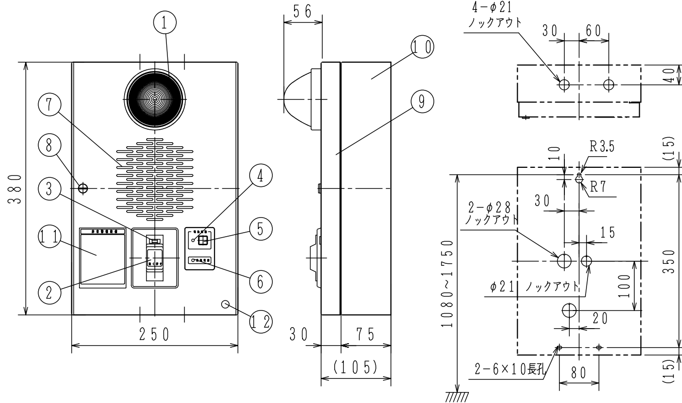
取付寸法図 (正面)
