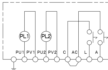
回路図
