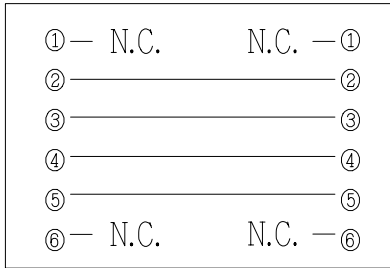
モジュラーケーブル結線図
