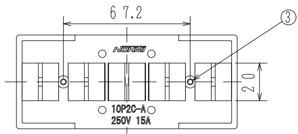
裏面図
