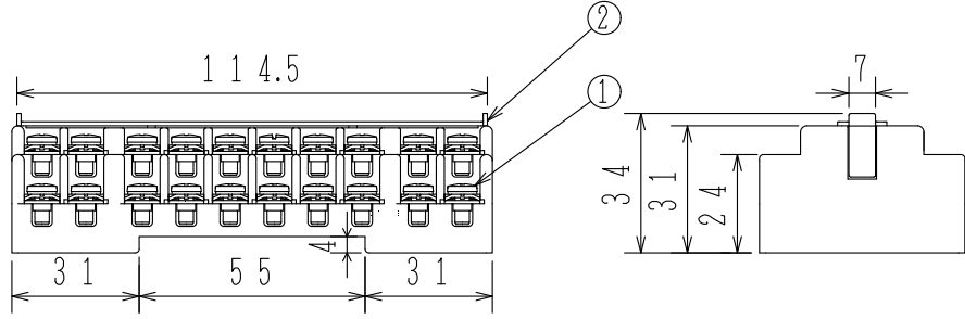
側面図
