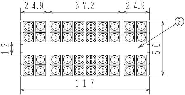
上面図
