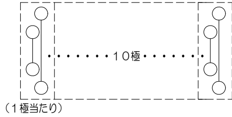
回路図
