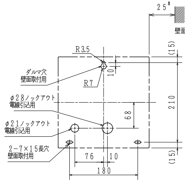
取付寸法図 (正面)
