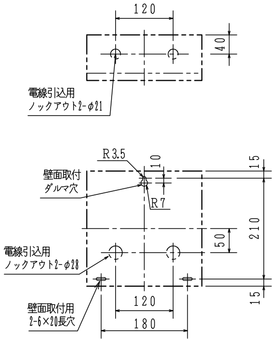
取付寸法図 (正面)
