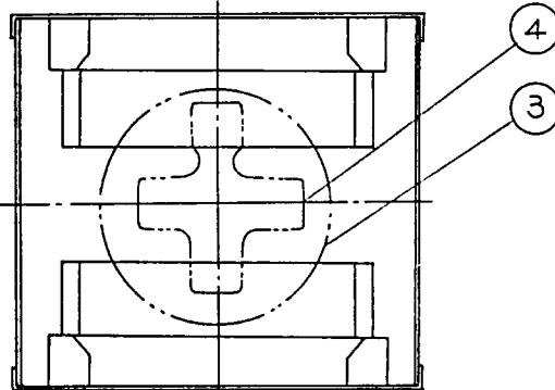
2) 電鈴取付図 (FXB 054型)
