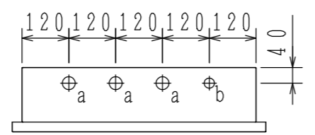
受信機組込図
