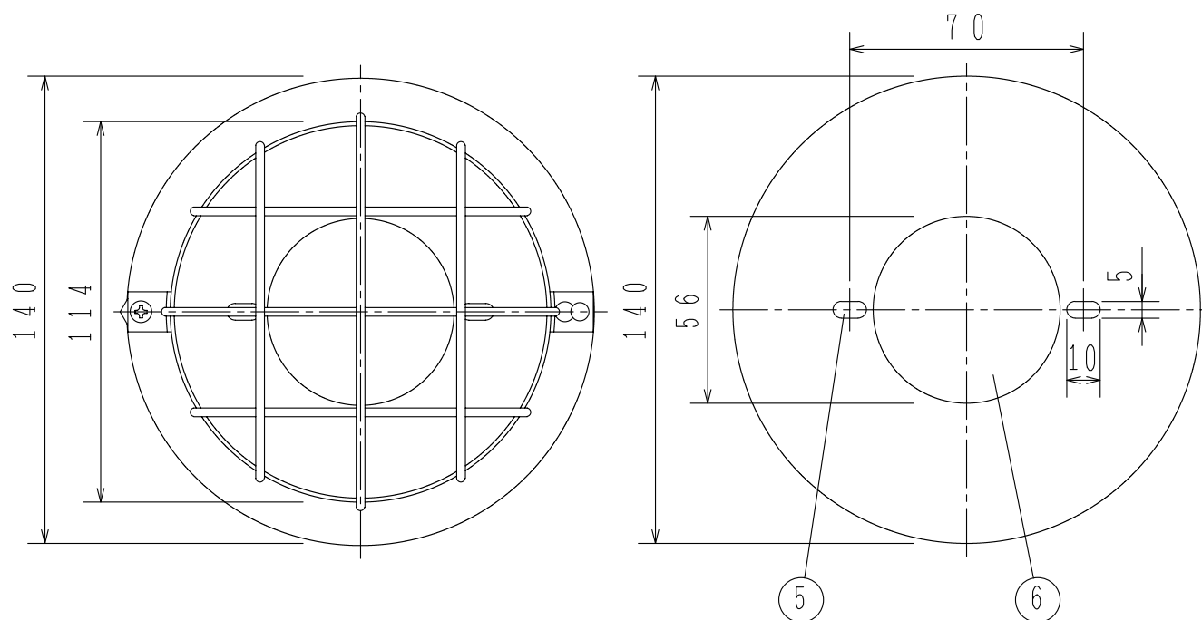
ベースプレート取付寸法図
