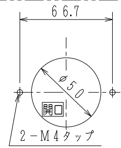
パネル加工図 (正面図)
