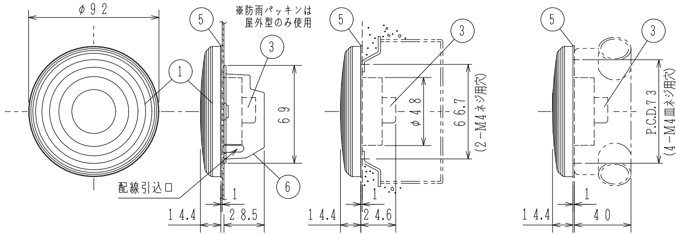
板金取付の場合
