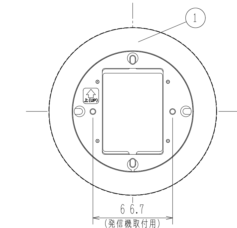
発信機アダプタプレート図 (正面図)
