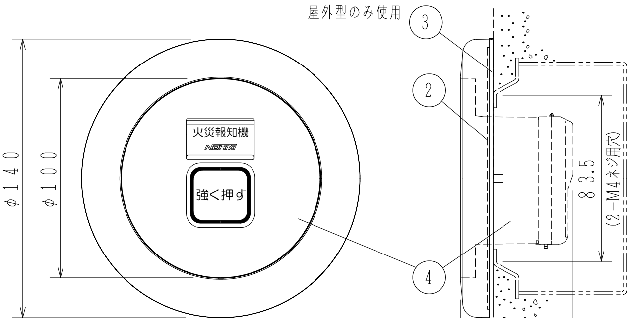
発信機組合せ例 (正面図)
