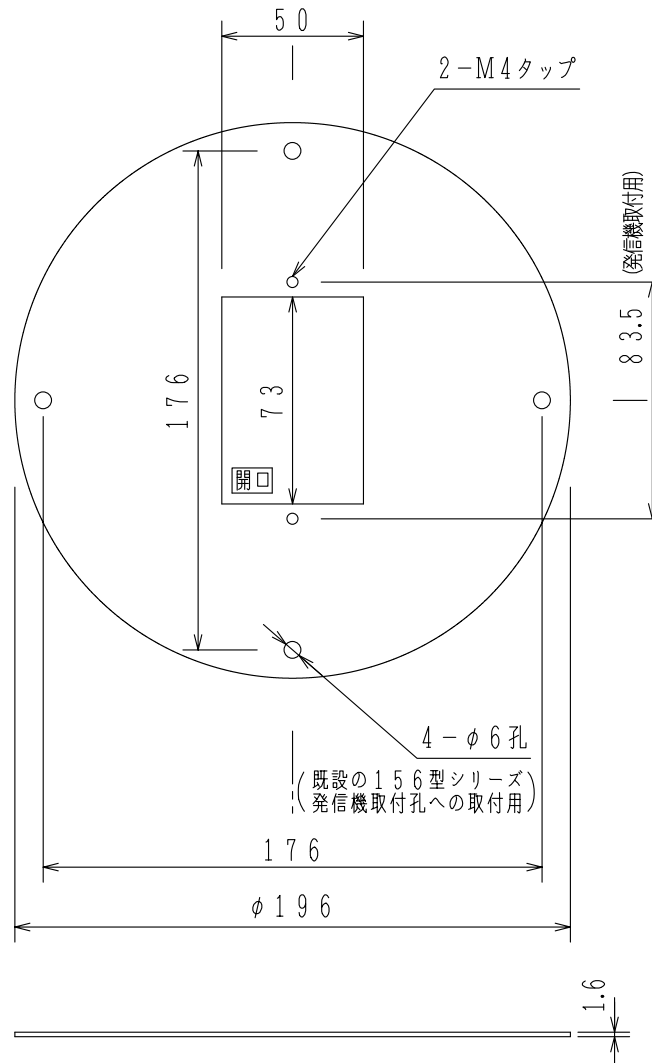
製作図
