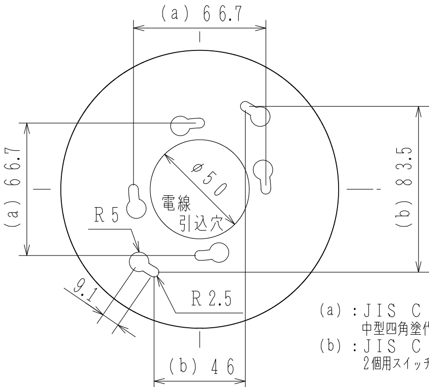
取付寸法図（正面図）
