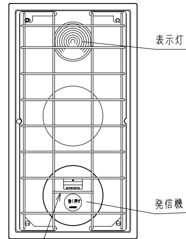
取付図
