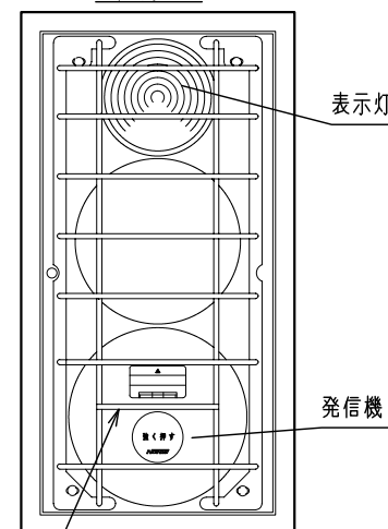
取付図
