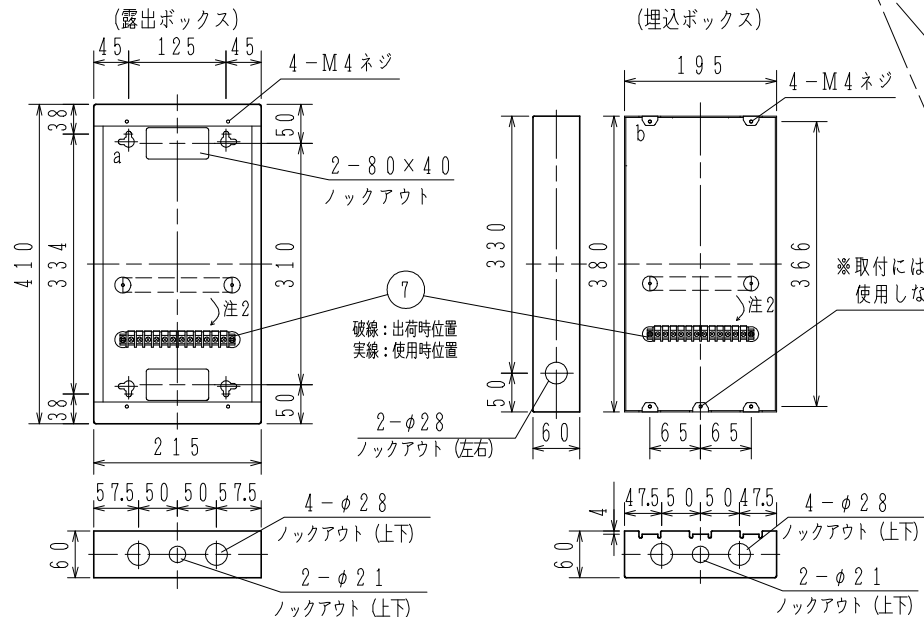
取付寸法図
