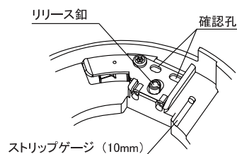
図 2. 端子部拡大図
