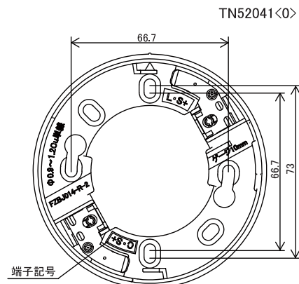
図 1. 取付寸法図
