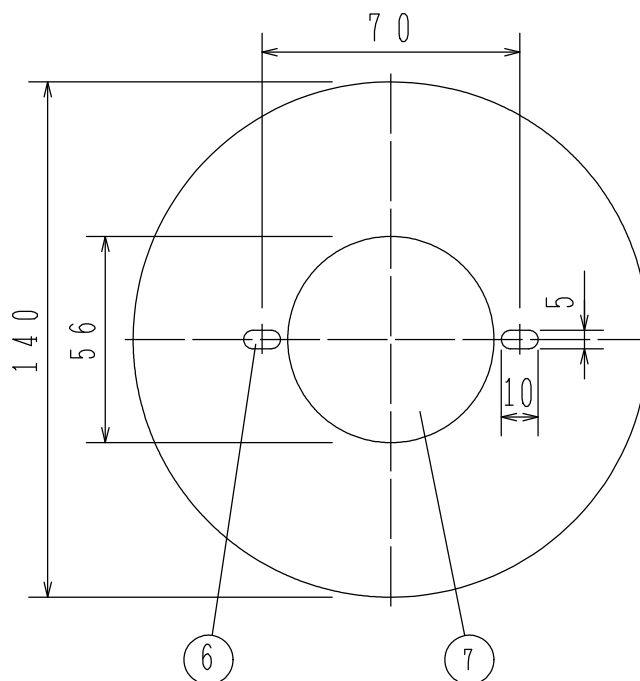
ベースプレート取付寸法図
