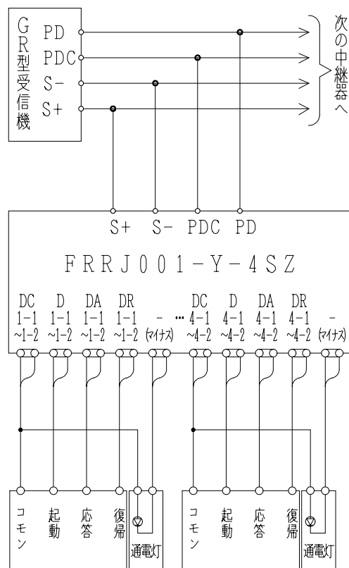
接続図
