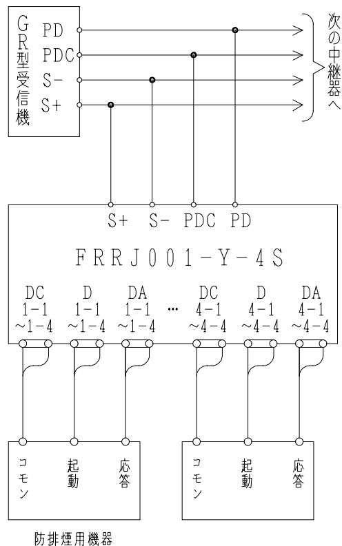
接続図
