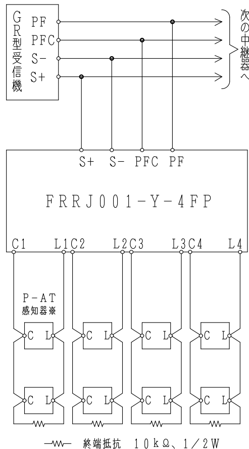
接続図
