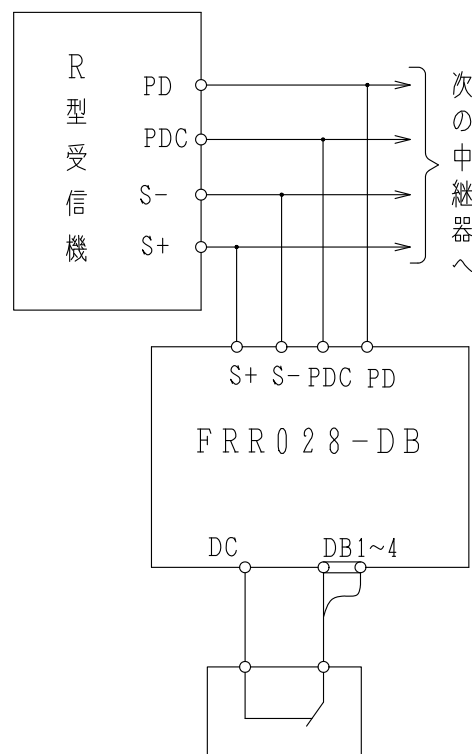
接 続 図
