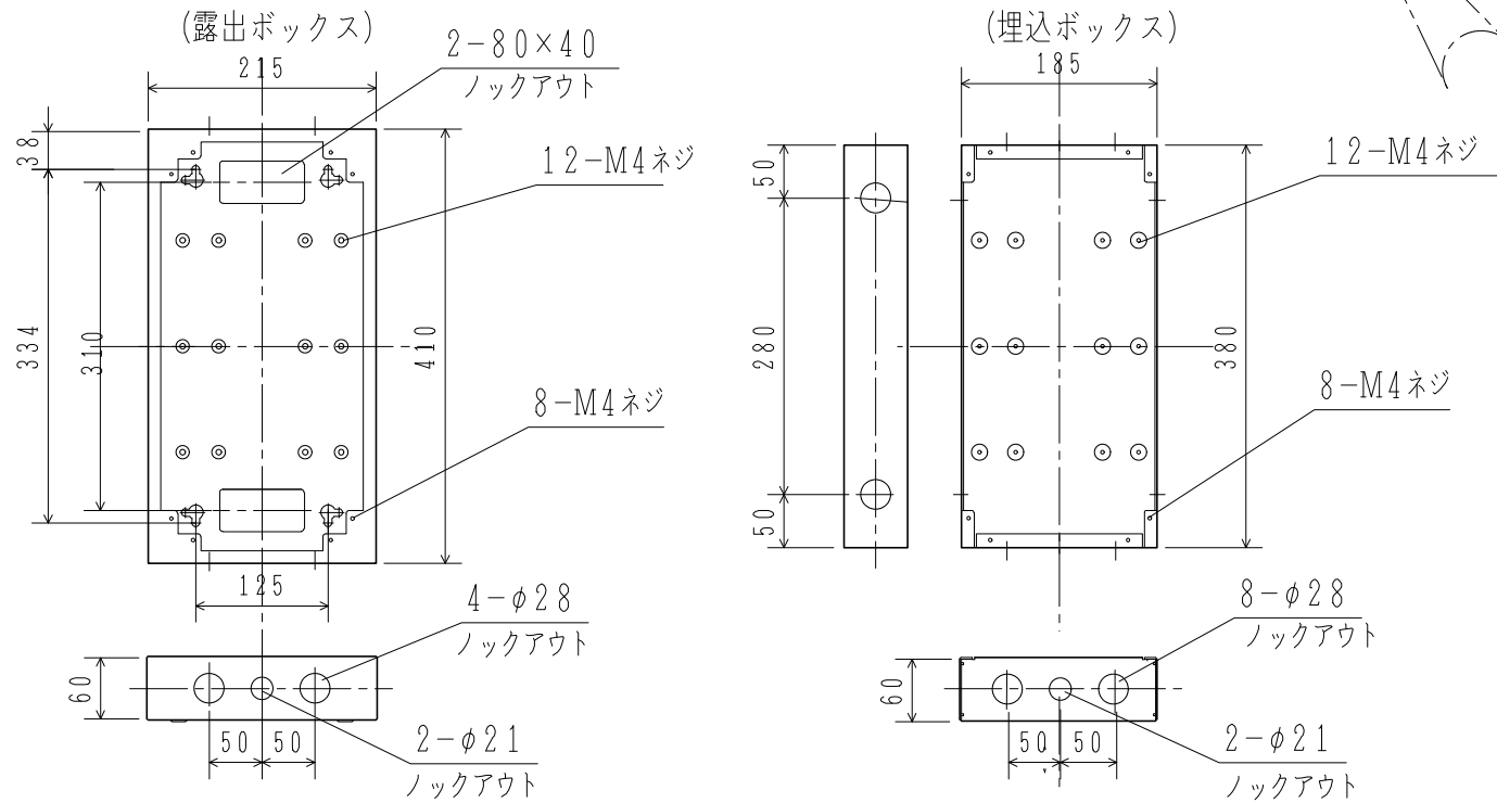
取付寸法図
