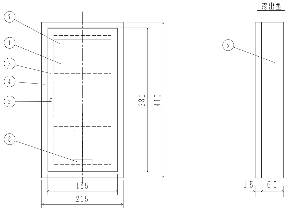
取付寸法図
