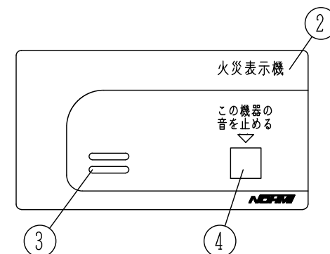
スイッチ操作部詳細図
