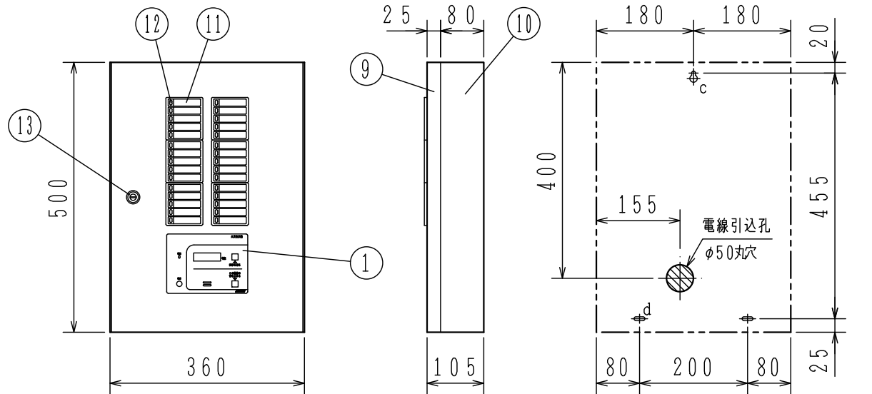
取付寸法詳細図（正面図）
