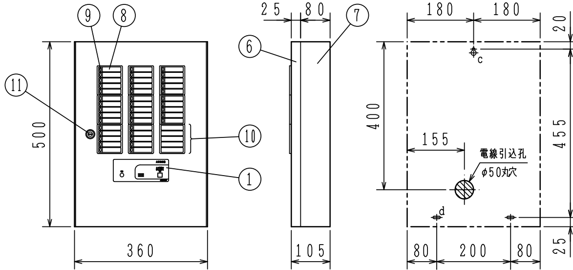
取付寸法詳細図 (正面図)
