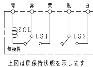
回路図
