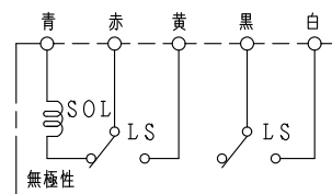
回路図
