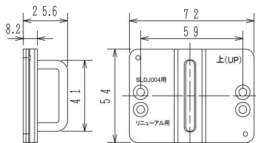
扉保持フック（防火戸へ取付）
